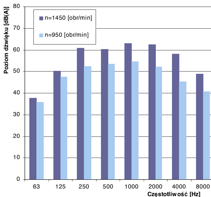
Poziomy dźwięku wentylatora WDC/sw 31,5-Ex dla poszczególnych częstotliwości
