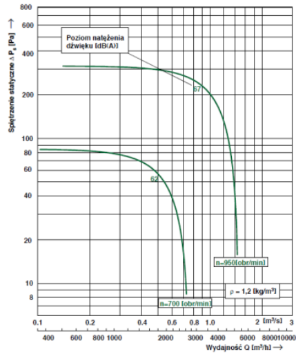
Charakterystyka przepływowa w wentylatora WKP 40-K
