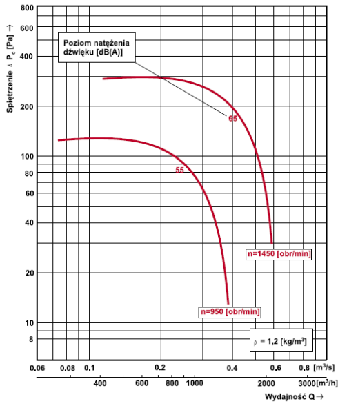
Charakterystyka przepływowa w wentylatora WKP 25-K
