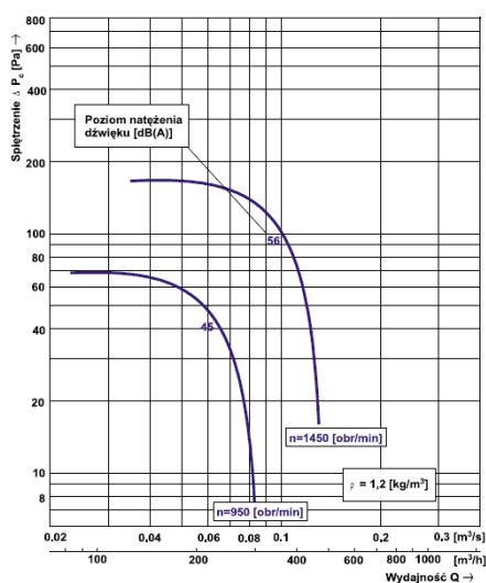
Charakterystyka przepływowa w wentylatora WKP 16-K
