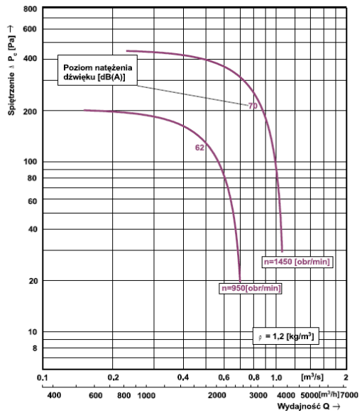
Charakterystyka przepływowa w wentylatora WKP 31,5-K
