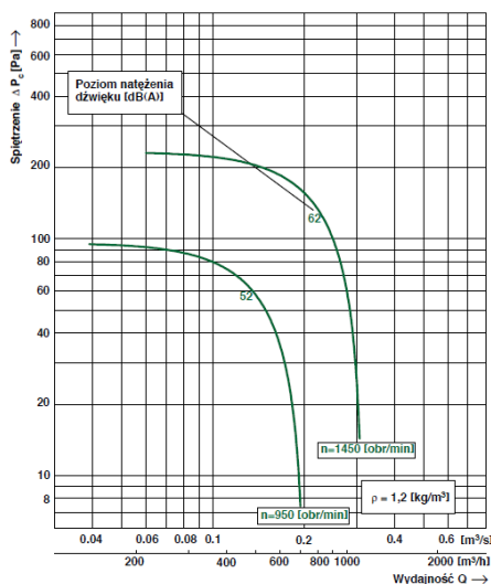
Charakterystyka przepływowa w wentylatora WKP 20-K
