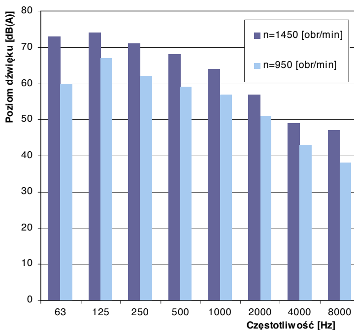
Poziomy dźwięku wentylatora WKP 31,5-K dla poszczególnych częstotliwości
