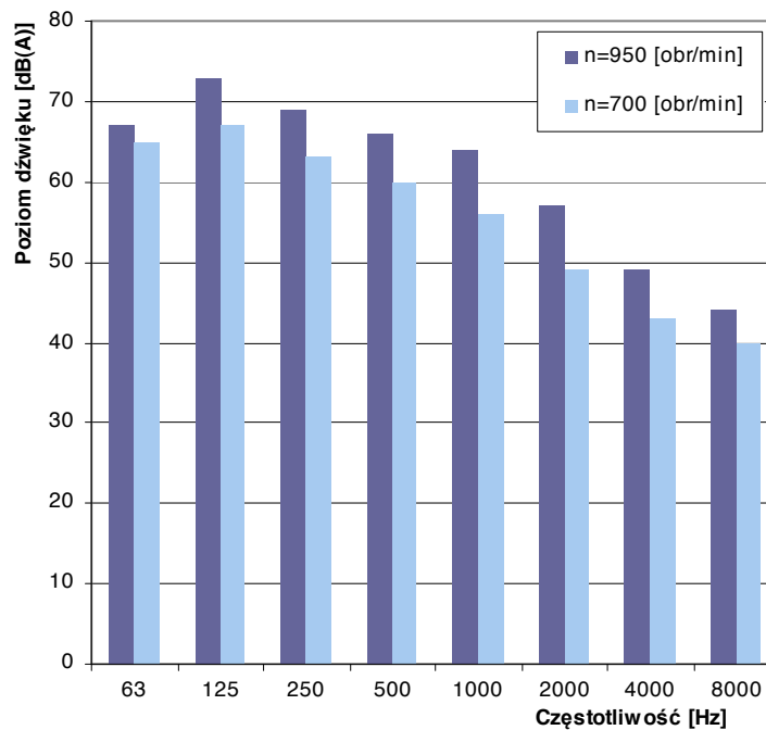
Poziomy dźwięk wentylatora WKP 40-K dla poszczególnych częstotliwości
